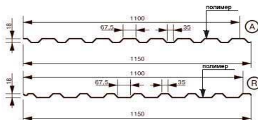
Профнастил тип П-20
